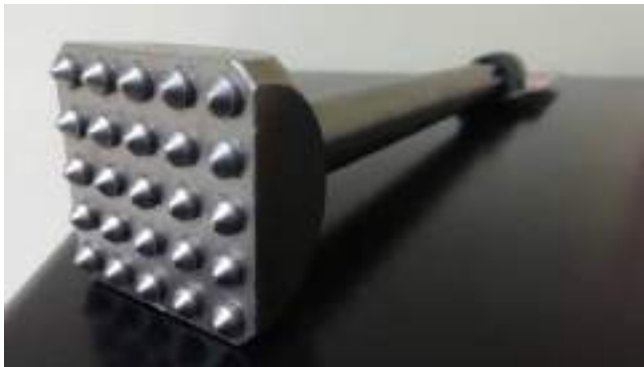
Bujarda de punta carburada SDS Max
